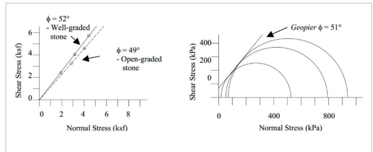
Figura 2. Ángulo de rozamiento en gravas usadas en Geopiers.
