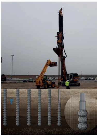
Figura 7. Columnas sistema Geopier Impact (Puerto de Tarragona).
