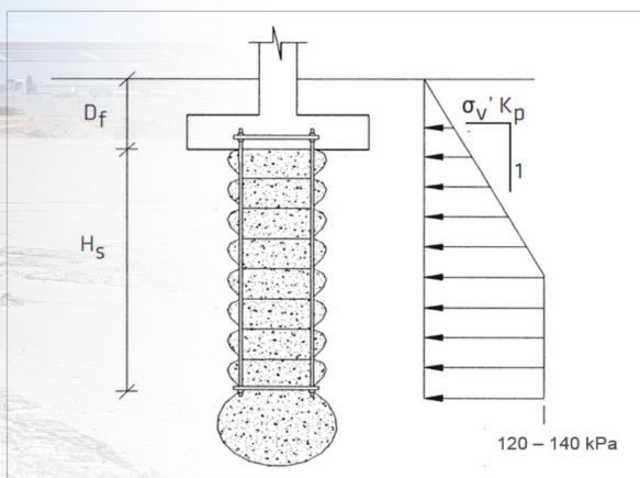
Figura 1. Empuje lateral generado al ejecutar columnas Geopier.
