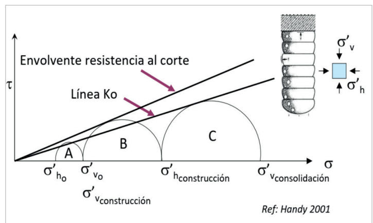
Figura 3. Efecto del pre-esfuerzo lateral en el aumento de resistencia al corte y capacidad portante.
